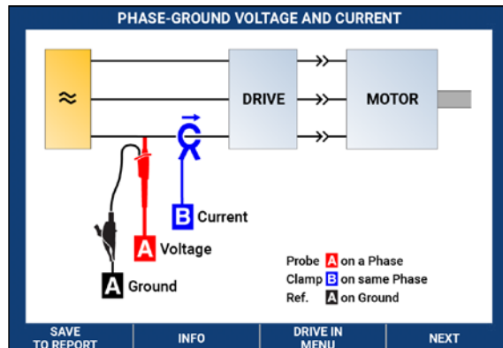
드라이브 입력 단계별 측정 연결 안내
