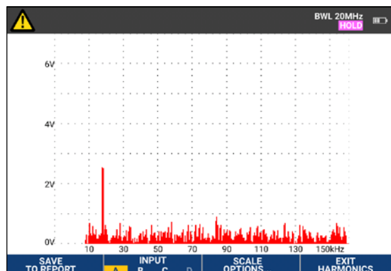
9kHz에서 150kHz로 확장된 고조파 스펙트럼
