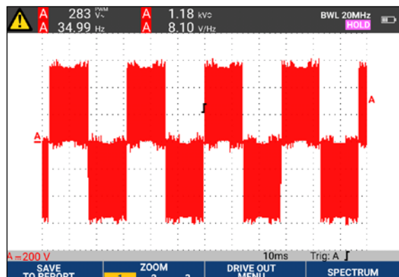
드라이브 출력 파형 자동 트리거
