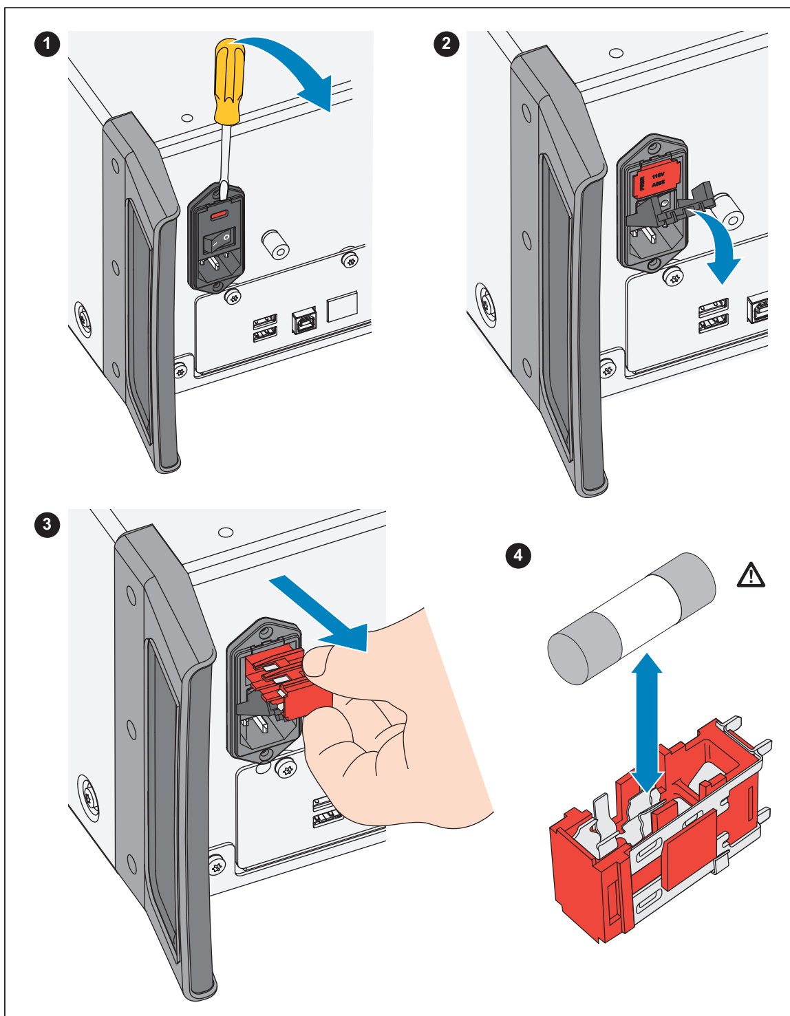
그림 15. 퓨즈에 접근
