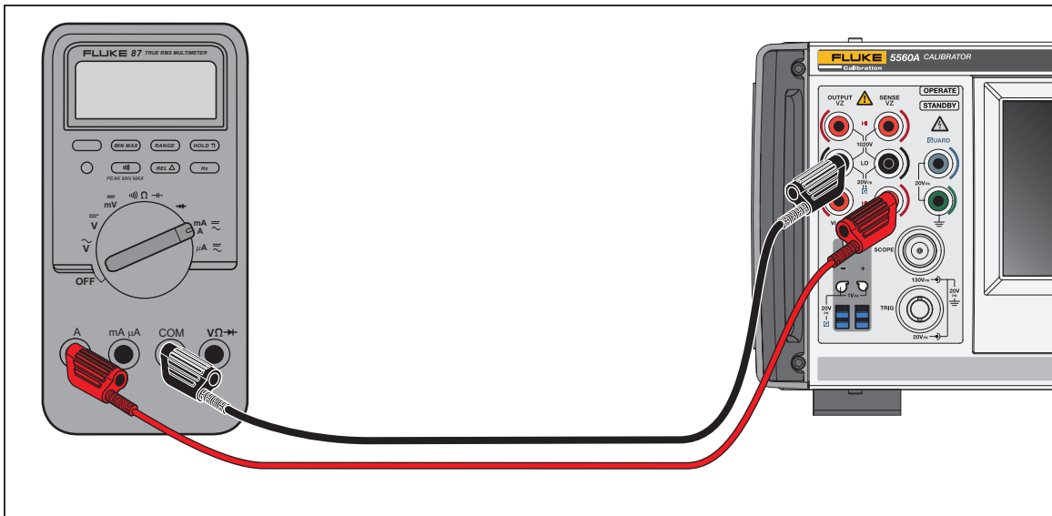
그림 8. DUT 연결 : DC 전류 / AC 전류 \geq 3.1 A
