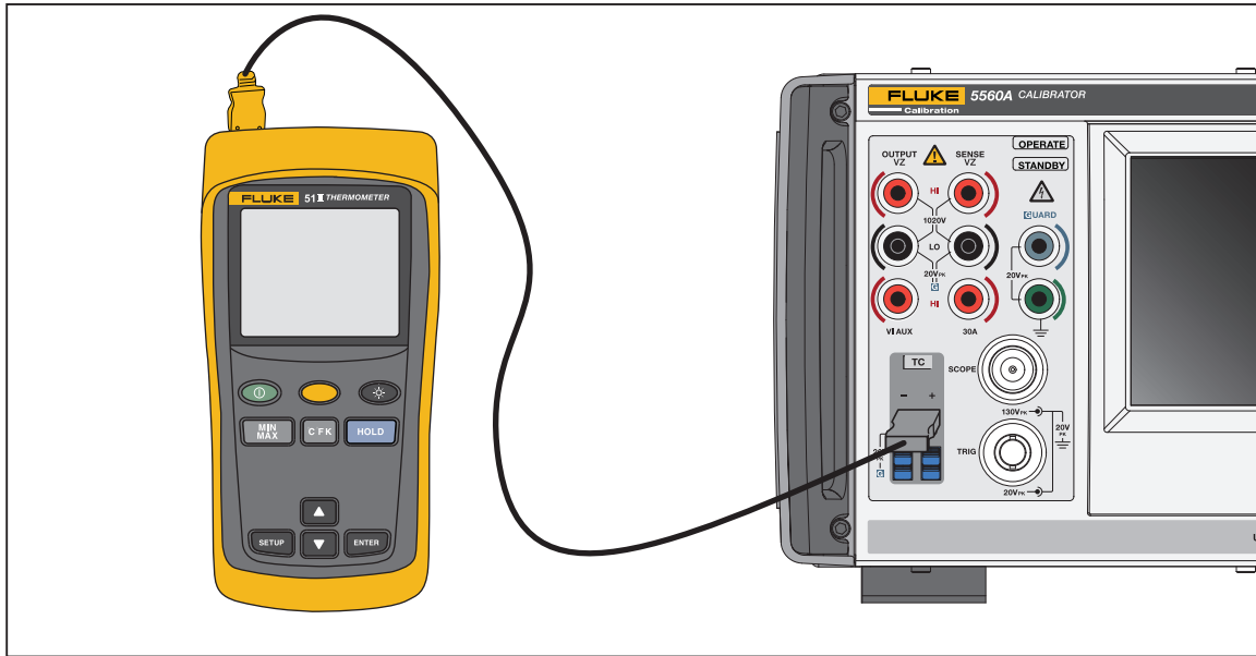
그림 14.50 시리즈 온도계 테스트를 위한 케이블 연결
