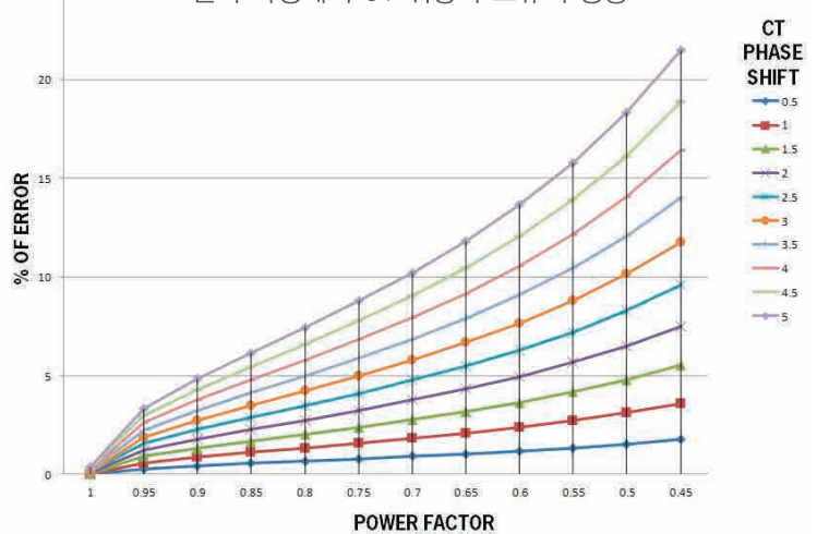
전력 측정에서 CT 위상각 오류의 영향
